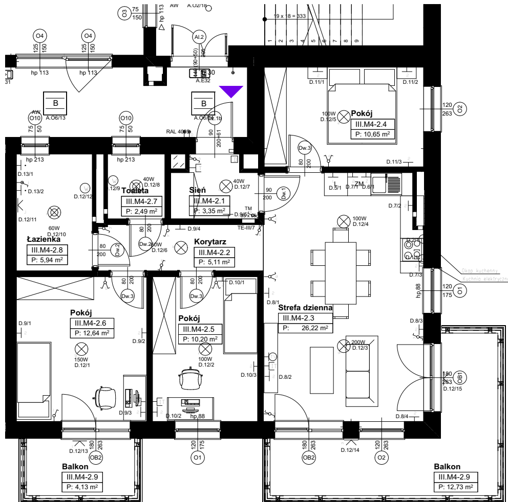
RZUT w skali 1:100
