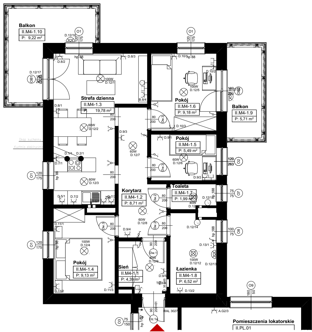
RZUT w skali 1:100
