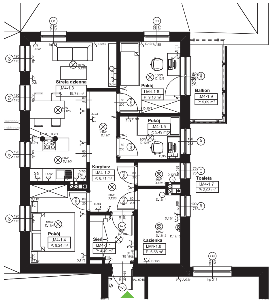
RZUT w skali 1:100
