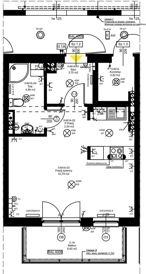
RZUT w skali 1:100
