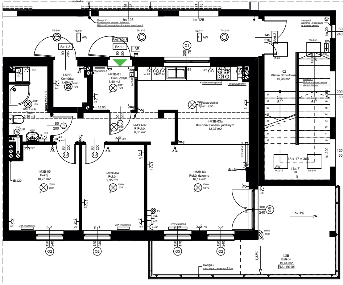
RZUT w skali 1:100
