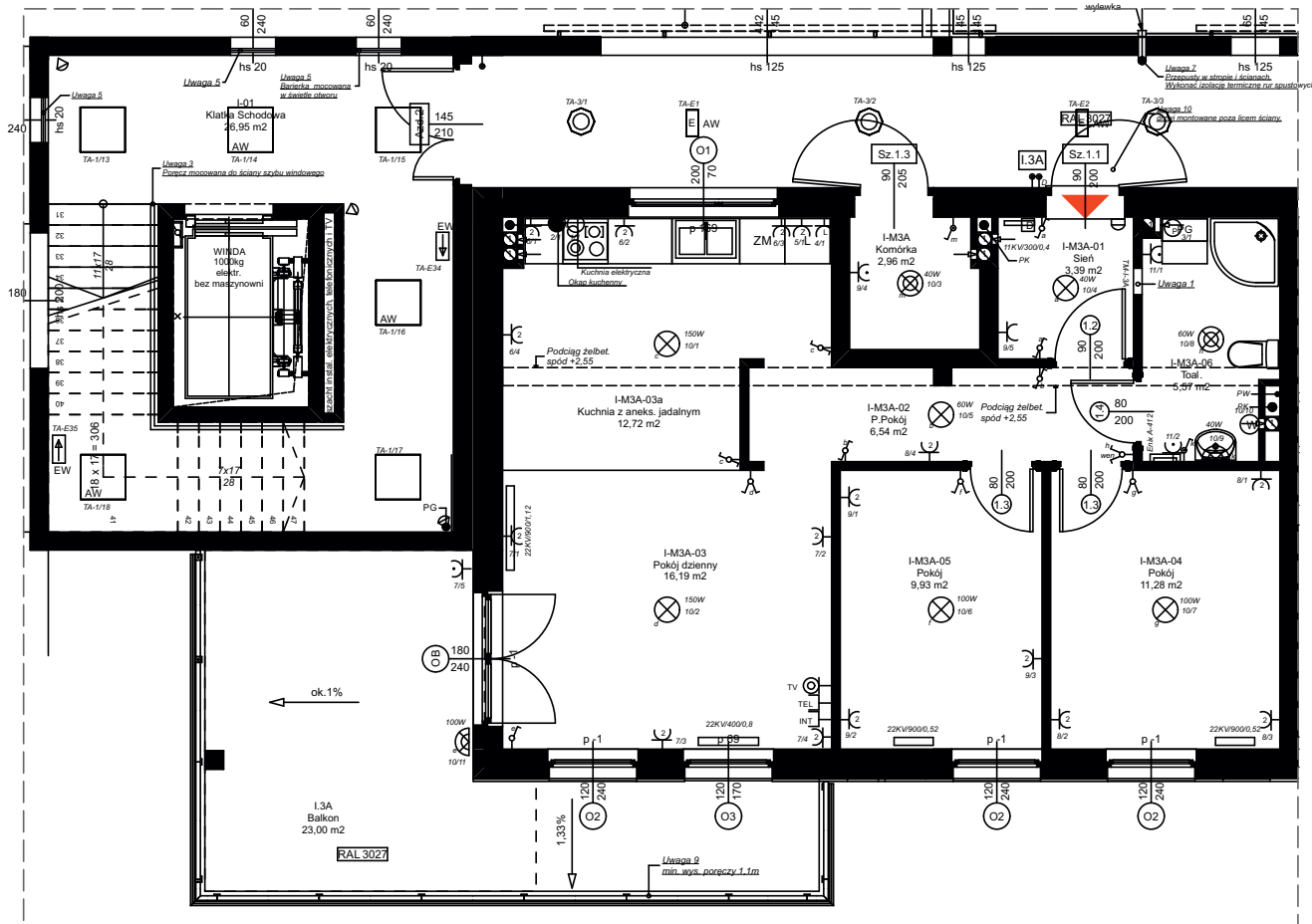
RZUT w skali 1:100
