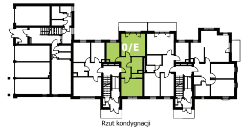
Rzut kondygnacji
